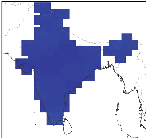
ECMWF
