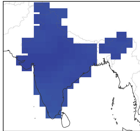
MME
