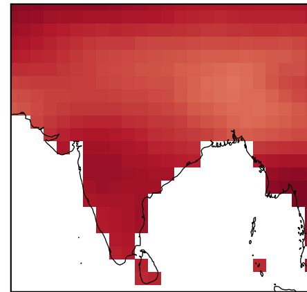
MME
