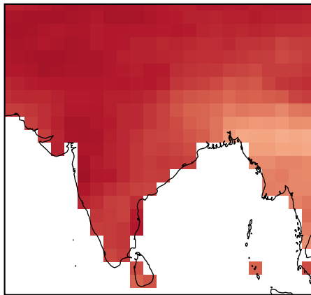
FuXi
