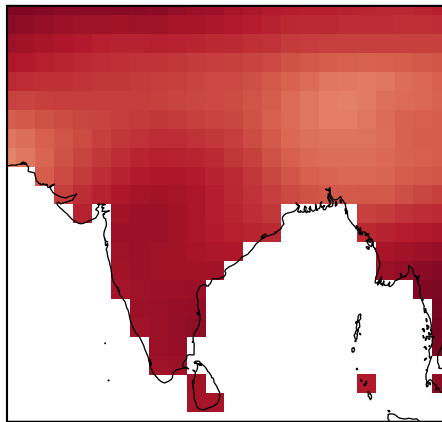
ECMWF
