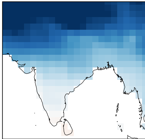
FuXi
