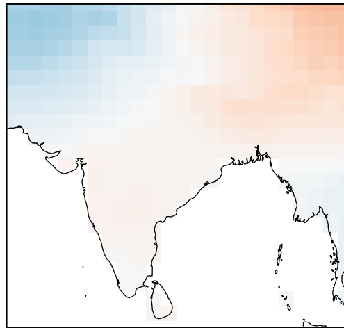
ECMWF
