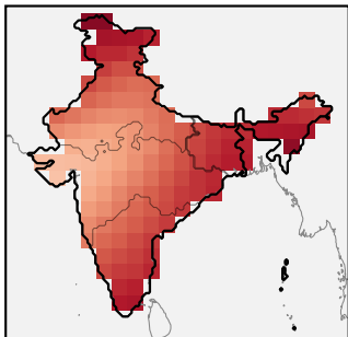
ECMWF
