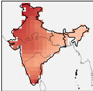
FuXi-S2S
