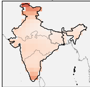
DLESyM
