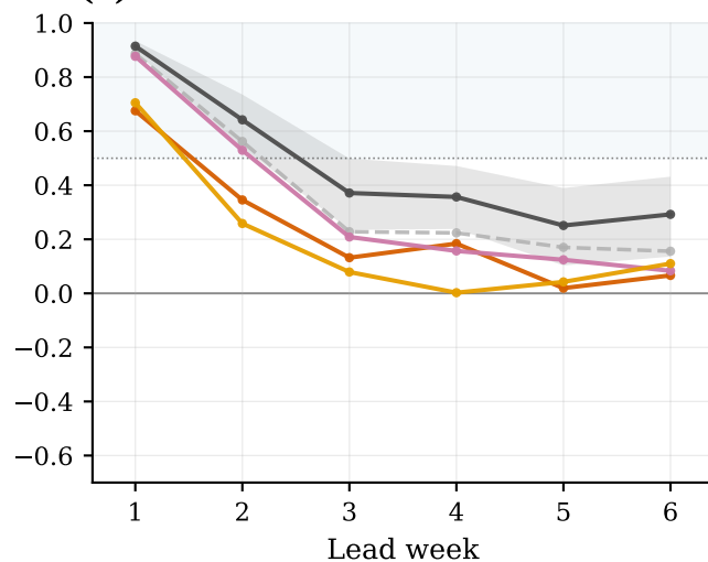
JJAS 2019 — Z500
