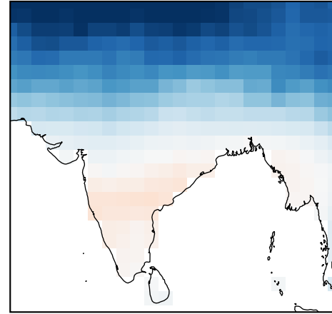
FuXi-S2S
