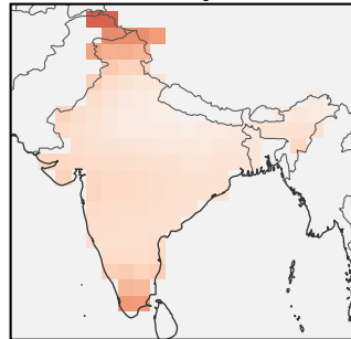
DLESyM
