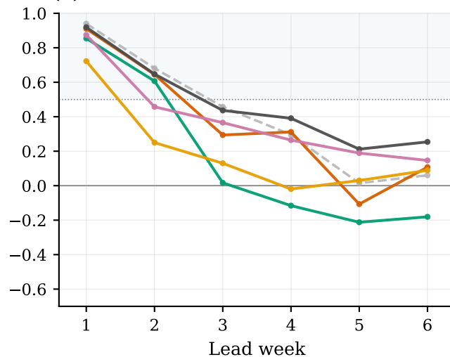
JJAS 2019 – Z500
