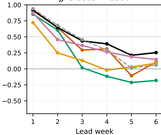
JJAS 2019 — Z500
