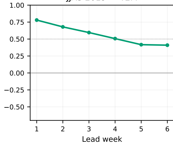
JJAS 2019 — T2M
