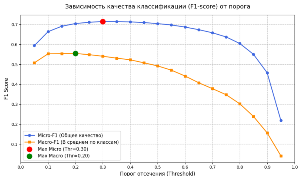
Рис. 2: Подбор порога
