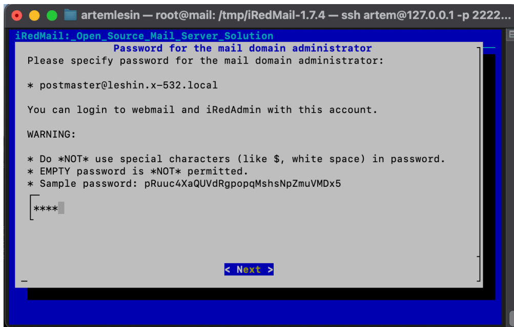
Рисунок 12 — Установка пароля почтового администратора
