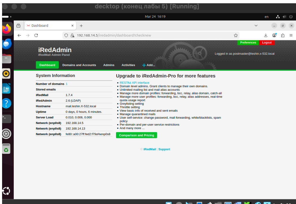
Рисунок 15 — Интерфейс iRedAdmin после входа
