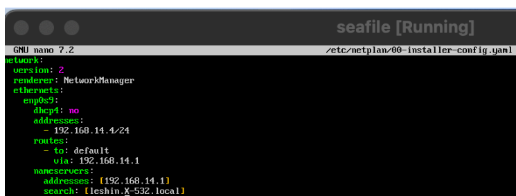
Рисунок 2 — Содержимое файла /etc/netplan/00-installer-config.yaml
