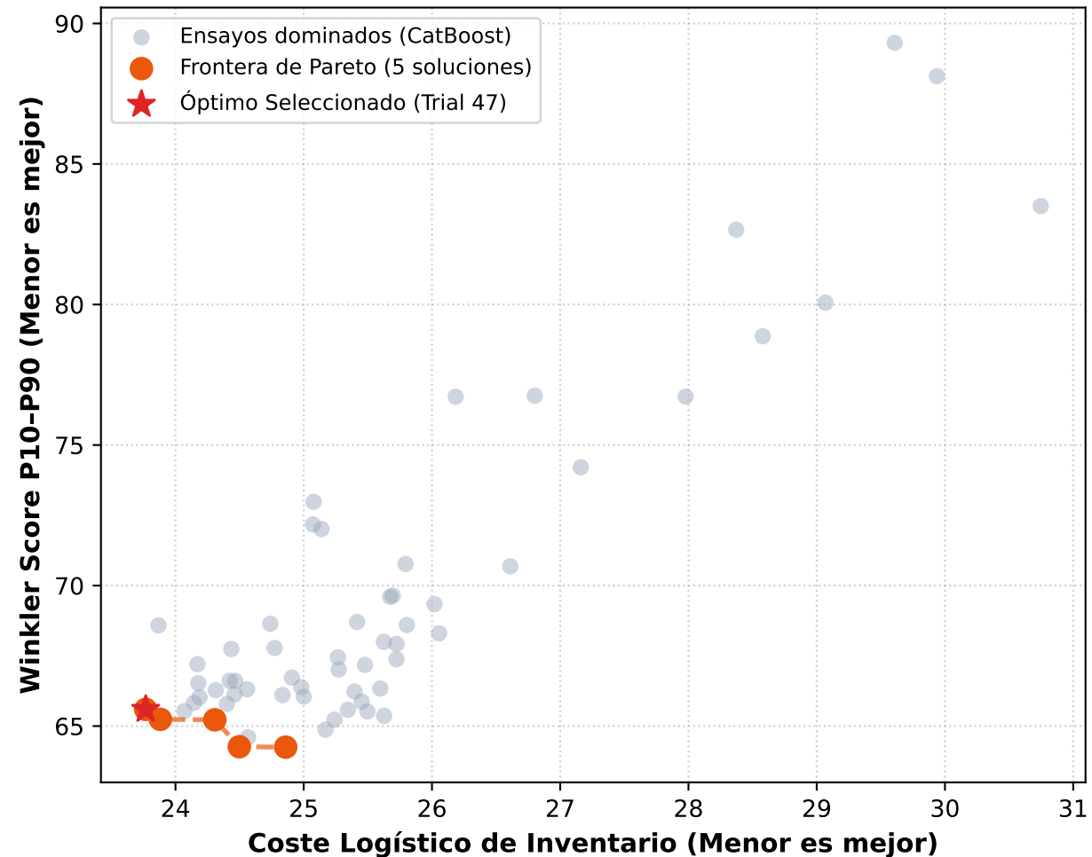
Frente de Pareto · CatBoost (60 Ensayos)
