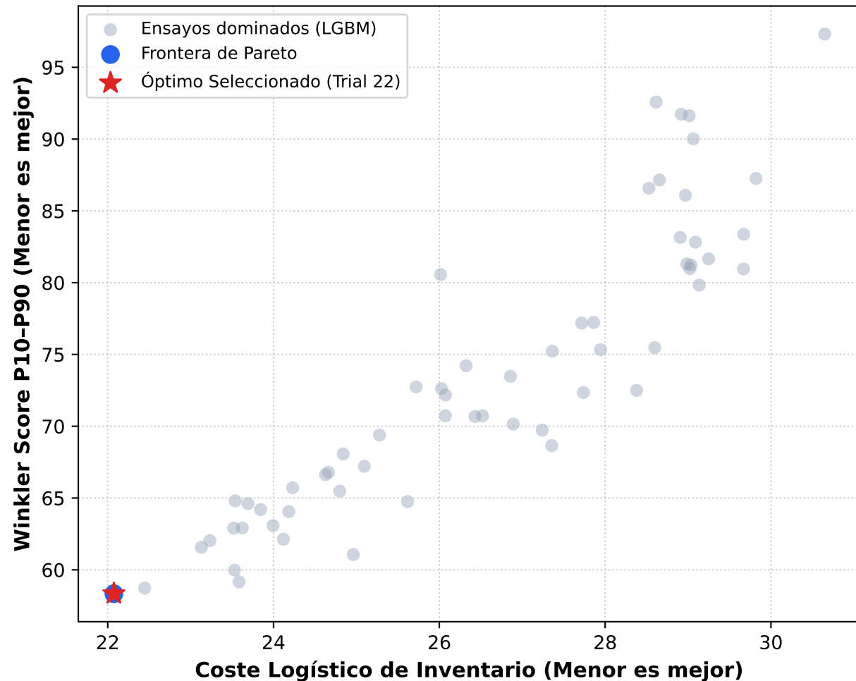
Frente de Pareto · LightGBM (60 Ensayos)
