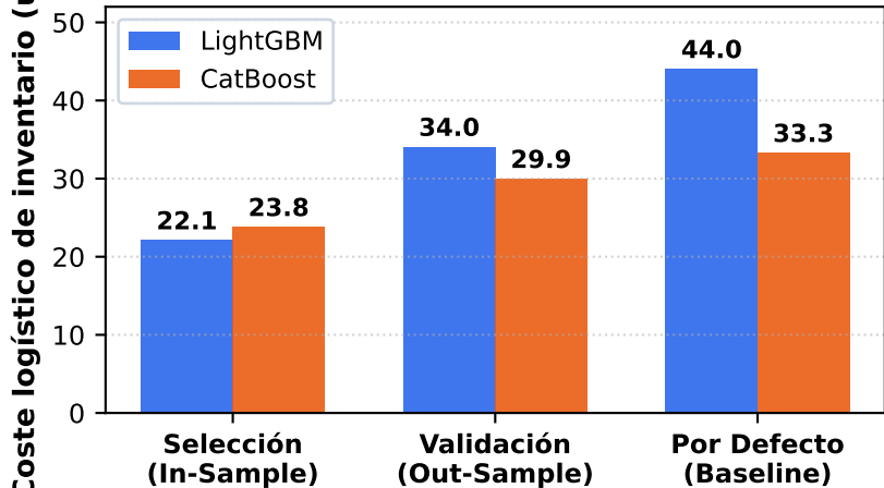
B. Estabilidad Fuera de Muestra ( N = 25 )
