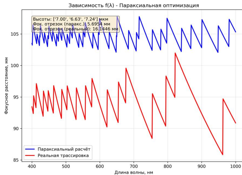
Рисунок 11 – Сравнительный анализ параксиального алгоритма и метода трассировки лучей 3х линз. Значения оптимальных высот соответствуют параксиальному случаю
