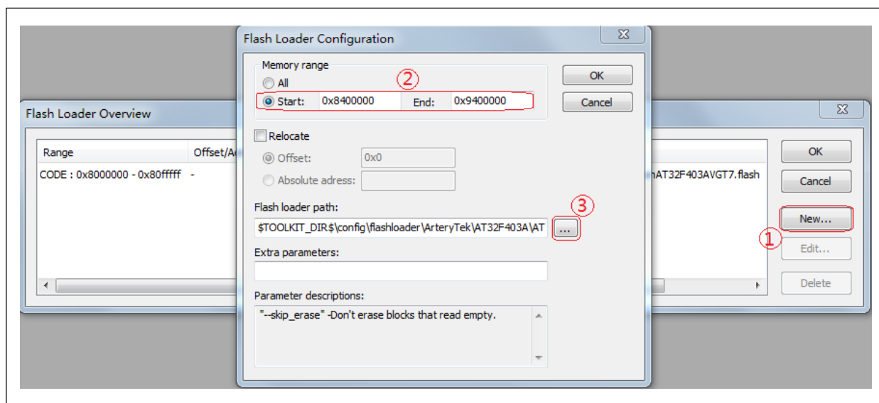
图 22. IAR Flash Loader 配置
