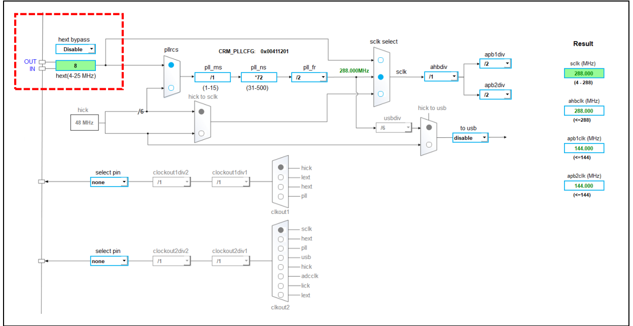
图 38. AT32_New_Clock_Configuration 界面
