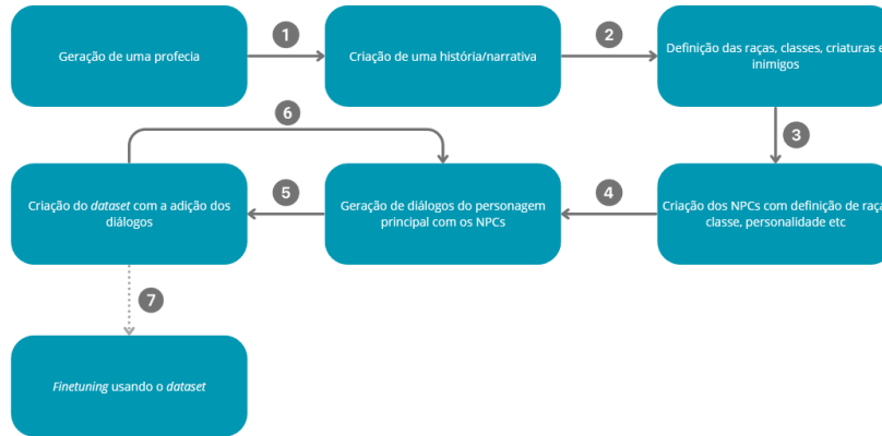
Figura 5.2: Fluxograma de Criação do Dataset de Treinamento
