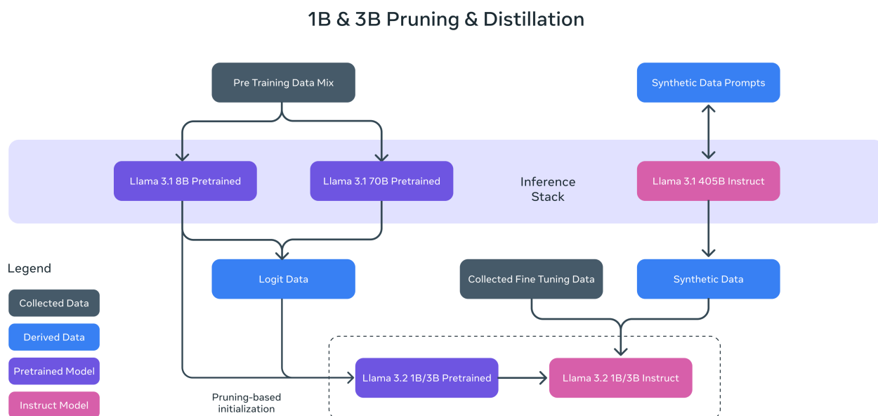
Figura 4.1: Processo de criação do Llama 3.2
