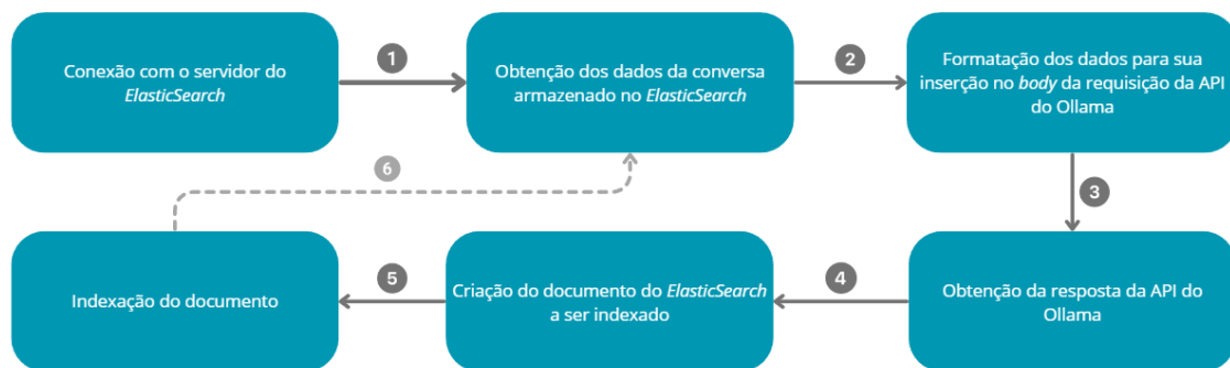
Figura 5.6: Fluxograma da Chamada da API
