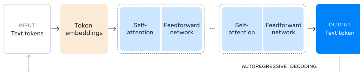
Figura 4.2: Arquitetura do Llama 3
