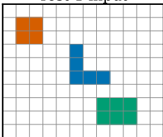
Test 1 input
