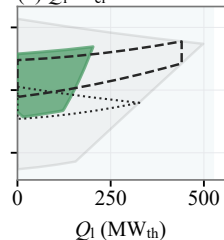
(d) Q_{\text{l}} \text{--} P_{\text{el}}
