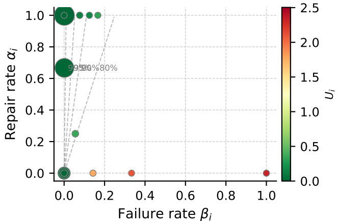
Markov Chain Parameters
