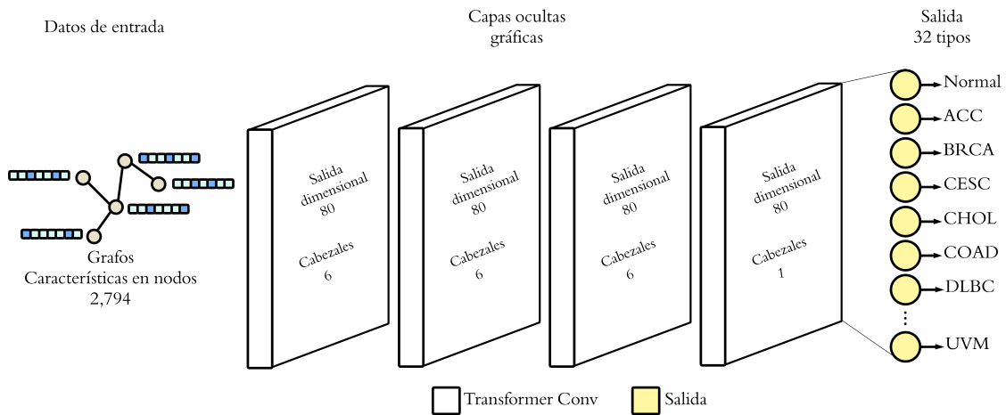
Figure 10: Arquitectura Graph Transformer (GTN). Diagrama del flujo de atención mediante bloques TransformerConv ( 80 \times 6 cabezales). A diferencia de los modelos piramidales, esta red mantiene una densidad constante de 480 dimensiones para el refinamiento de características globales. Se detalla la transición desde la entrada ( N = 2,794 ) hasta la salida de 32 clases, integrando Dropout de 0.5 y activaciones LeakyReLU.
