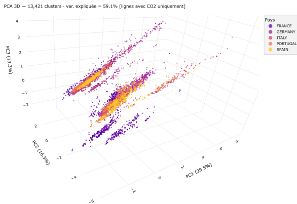
FIG. 9. Projection PCA (trois composantes, \approx 60\% de variance) et centroïdes k -means par marché : des clusters distincts apparaissent.
