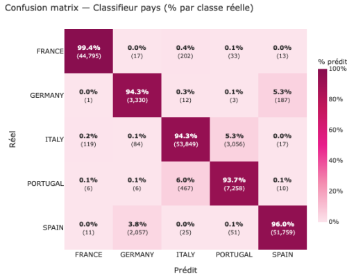
FIG. 8. Matrice de confusion du classifieur de domaine. Les marchés sont identifiés avec une grande fiabilité.
