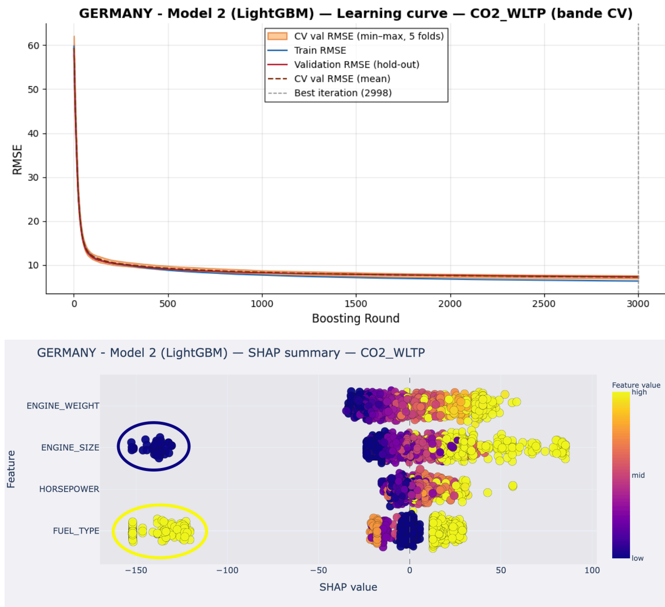
FIG. 5. Model 2 (light-scope), Allemagne, cible WLTP. Haut : learning curve ; bas : beeswarm SHAP. Overfitting jugulé, contributions directionnelles et lisibles (cluster électrique net sur FUEL_TYPE et ENGINE_SIZE).
