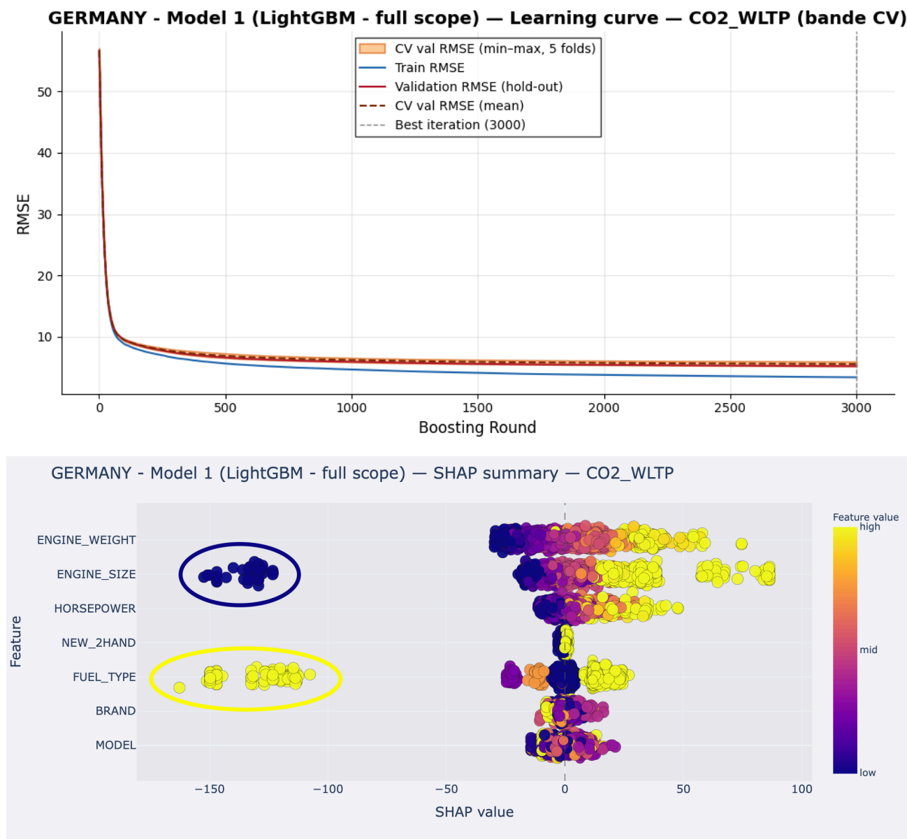
Fig. 4. Model 1 (full-scope), Allemagne, cible WLTP. Haut : learning curve ; bas : beeswarm SHAP. Overfitting visible ; BRAND, MODEL, NEW_2HAND présentent des contributions SHAP ramassées et non directionnelles.
