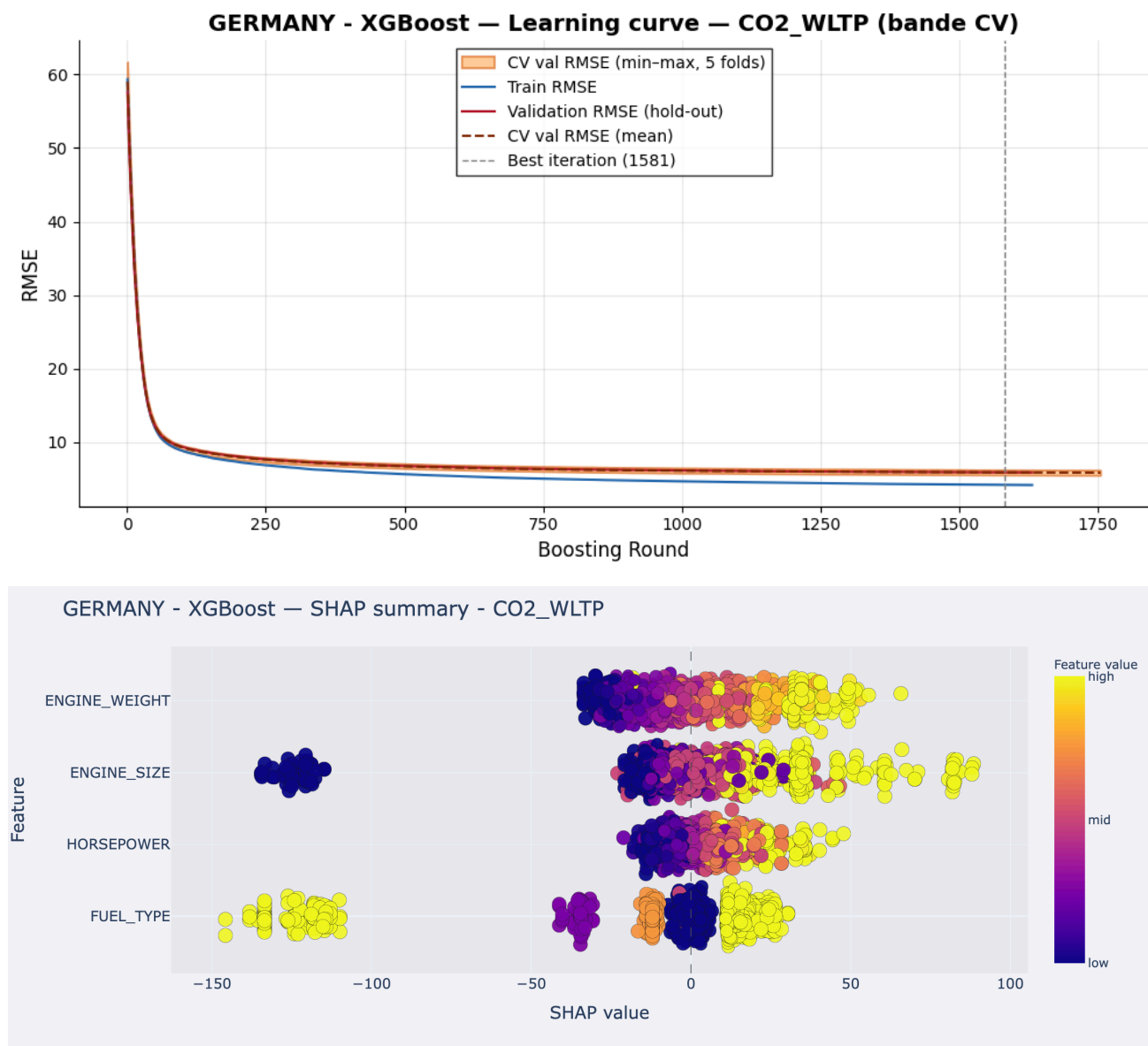
FIG. 6. XGBoost (light-scope), Allemagne, cible WLTP. Haut : learning curve ; bas : beeswarm SHAP. RMSE finale plus basse, mais overfitting réintroduit.
