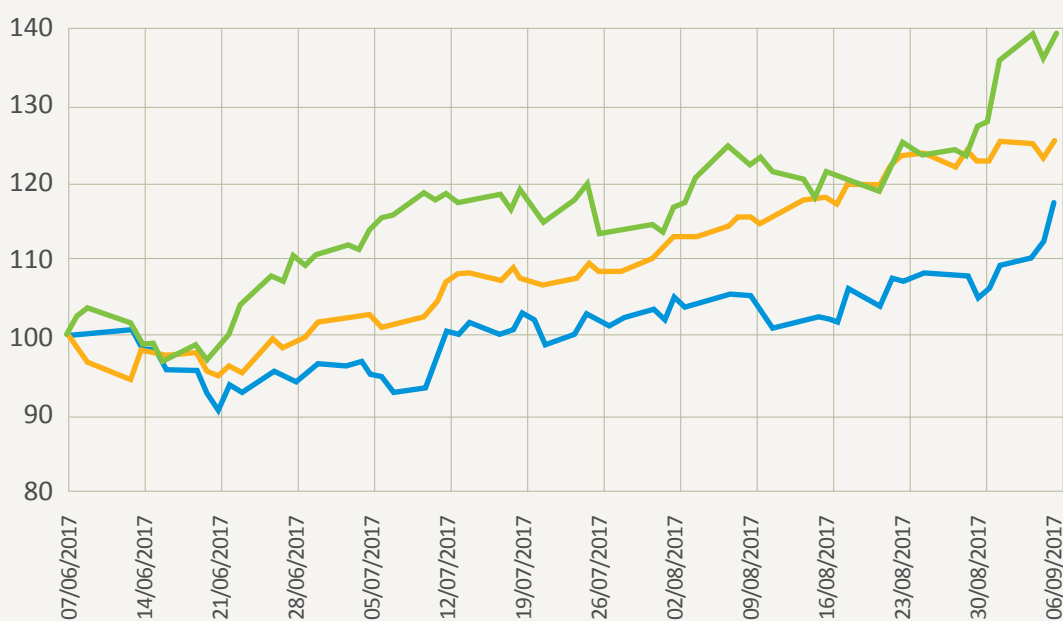
Gráfico 3. Desempenho das ações PETR4, BBDC4 e GGBR4 –normalizado – 7 de junho de 2017 a 6 de setembro de 2017
