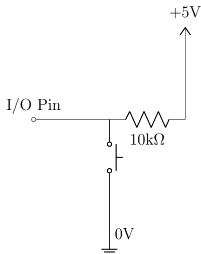
Figura 1: Exemplo Circuito
