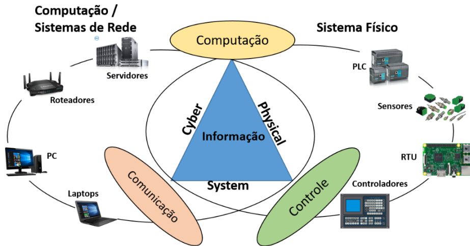
Figura 3: Estrutura de um Sistema Ciber-Físico
