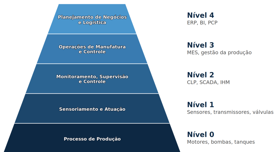
Figura 2: Pirâmide de Automação
