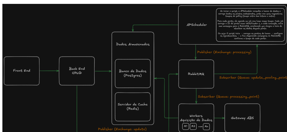
Figura 7: Arquitetura do Sistema
