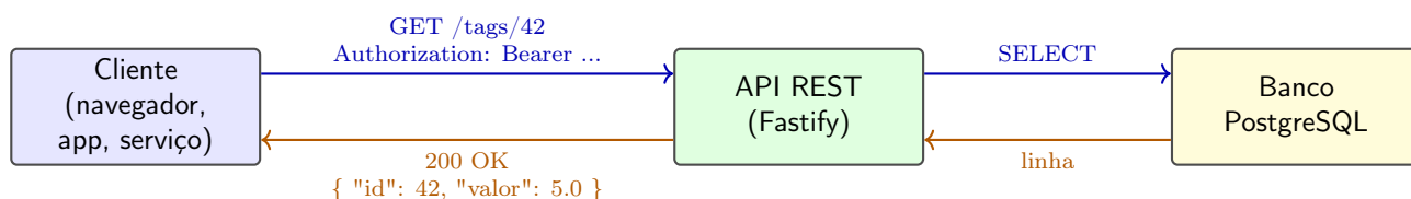
Figura 15: Ciclo requisição-resposta HTTP em uma API REST
