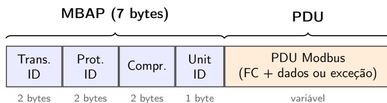
Figura 18: Composição lógica do Modbus TCP: cabeçalho MBAP seguido da PDU (código de função, dados ou exceção)
