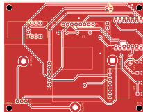
Cara Top (Display/ECG)
