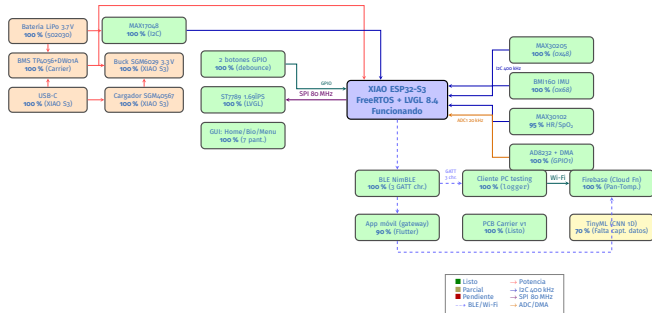
Figura: Arquitectura de hardware y estado de avance integrado para la Entrega 3.
