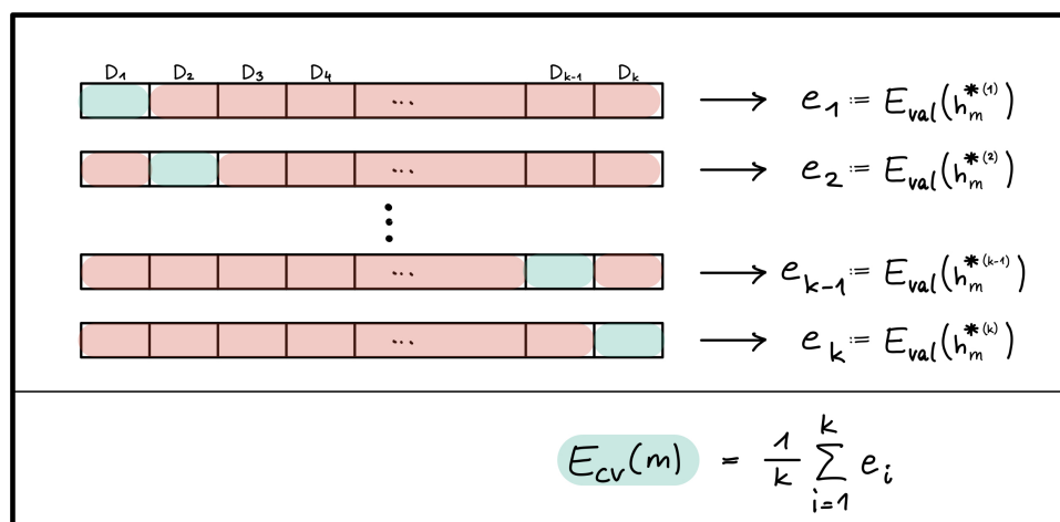
Abbildung 6.6.: Abbildung 4 - Kreuzvalidierung
