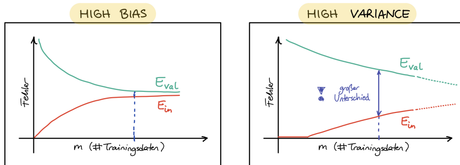
Abbildung 6.5.: Abbildung 3 - Lernkurven
