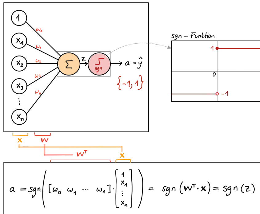
Abbildung 6.1.: Perzeptron Aufbau und Berechnung
