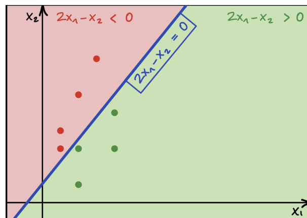
Abbildung 9.2.: Perzeptron Entscheidungsgrenze
