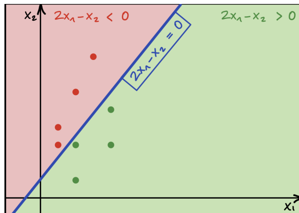
Abbildung 6.2.: Perzeptron Entscheidungsgrenze
