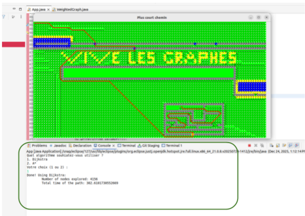
Figure 2 - Visualisation du chemin rouge tracé par Dijkstra sur la carte
