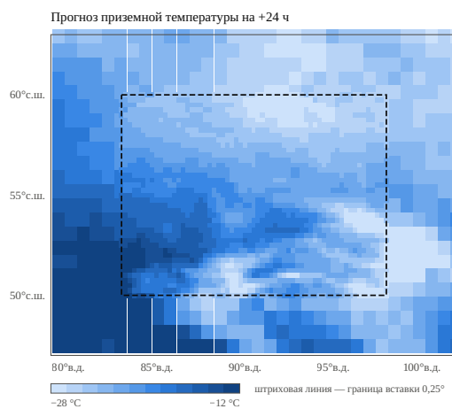
Рис. 1. Прогноз приземной температуры на +24 ч в окрестности границы региональной вставки. Размер ячейки соответствует шагу сетки — 0,25° внутри вставки и 0,703° снаружи; штриховая линия — граница вставки.
