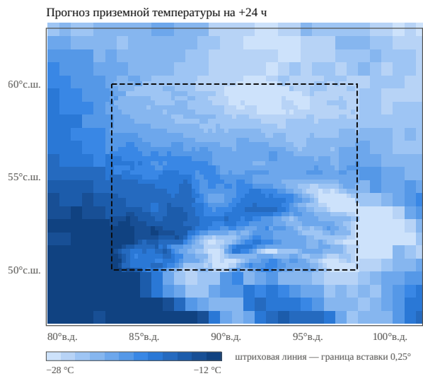
Рис. 2. Прогноз приземной температуры на +24 ч в окрестности границы региональной вставки. Размер ячейки соответствует шагу сетки — 0,25° внутри вставки и 0,703° снаружи; штриховая линия — граница вставки.
