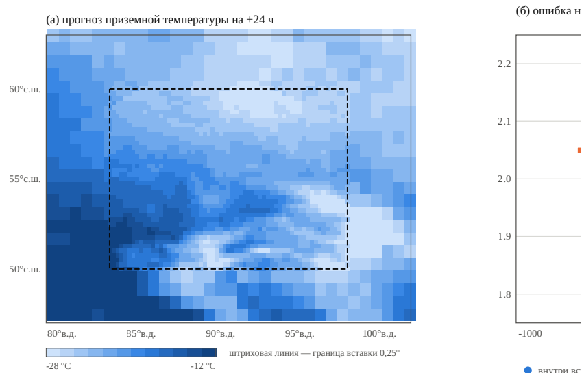
Рис. 2. Прогноз приземной температуры на +24 ч в окрестности границы региональной вставки. Размер ячейки соответствует шагу сетки — 0,25° внутри вставки и 0,703° снаружи; штриховая линия — граница вставки.
