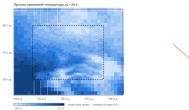
Рис. 1. Прогноз приземной температуры на +24 ч в окрестности границы региональной вставки. Размер ячейки равен шагу сетки: 0,25° внутри вставки и 0,703° снаружи. Штриховой линией показана граница вставки.
