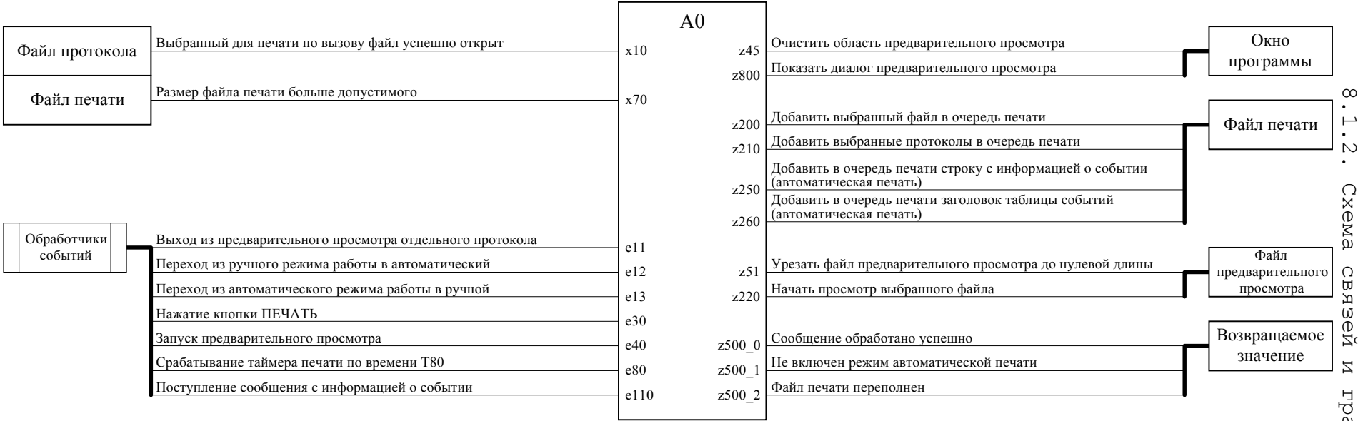
Автомат контроля режима печати. Схема связей автомата
