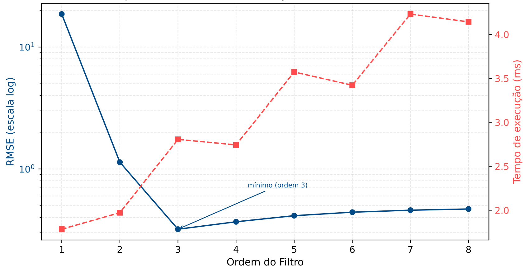
Custo Computacional vs. Ordem (Chebyshev II Fase Zero, f_c = 2700 Hz)
