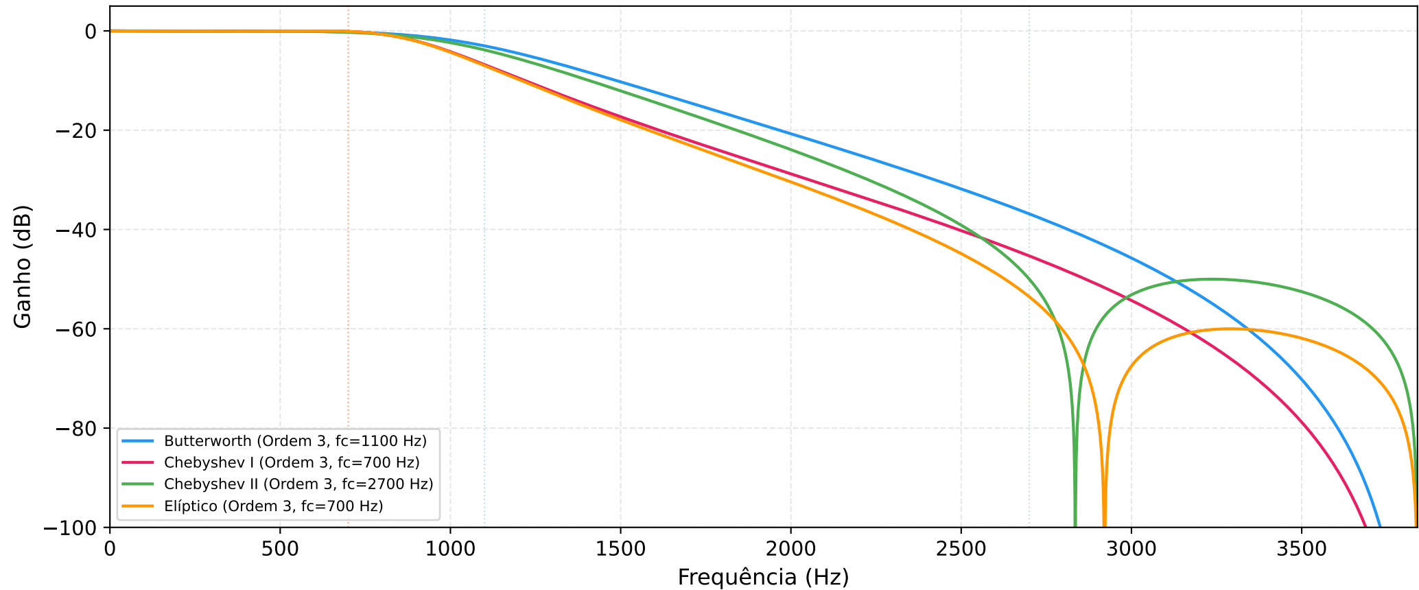
Resposta em Frequência dos Melhores Filtros
