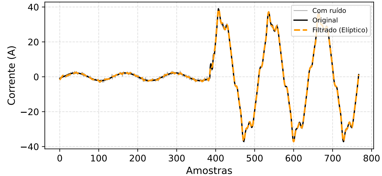
Elíptico — Ordem 3 | f_c = 700 Hz RMSE = 0.3262 | \Delta SNR = 5.2 dB
