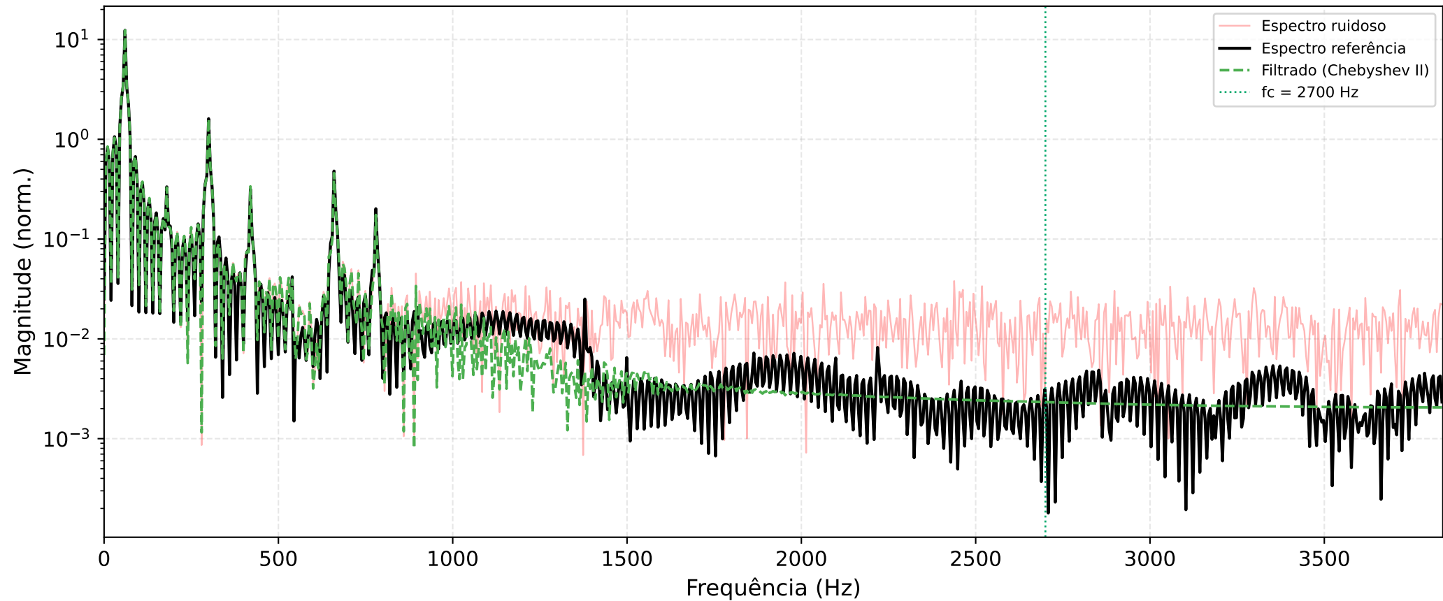
Espectro de Frequência — Antes e Depois da Filtragem
