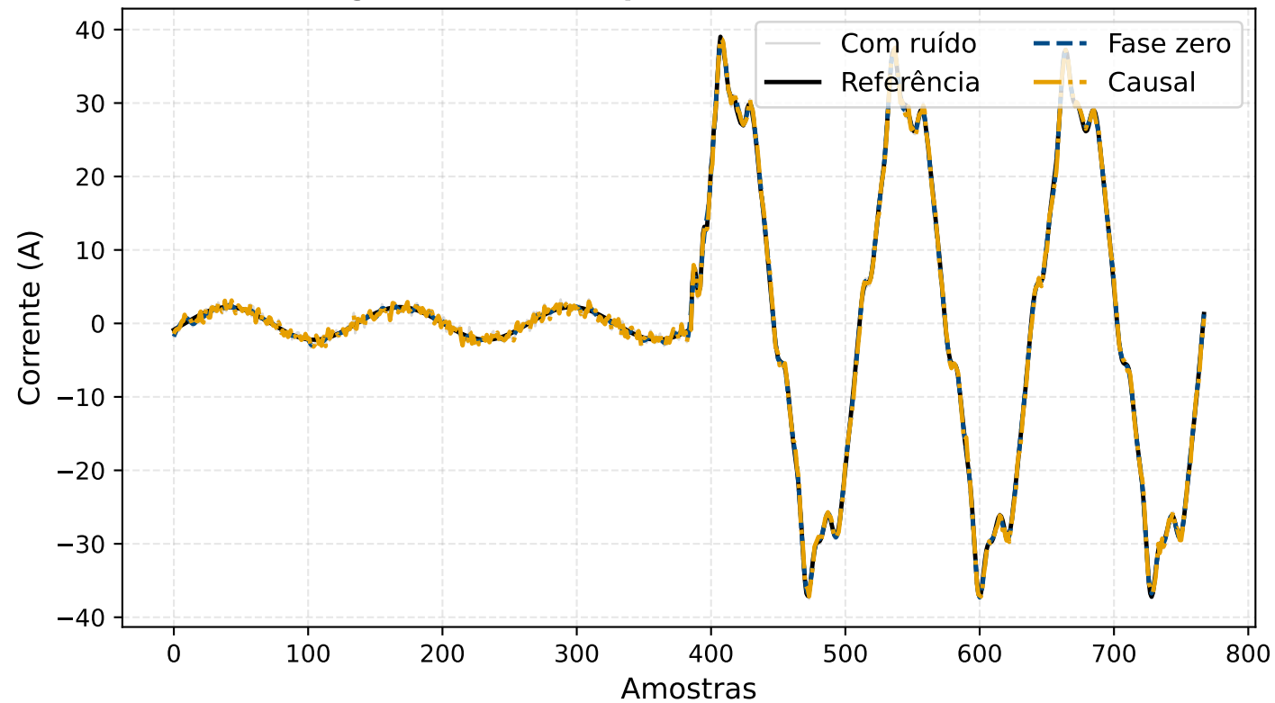
Filtragem Causal (tempo real) vs. Fase Zero (offline)
