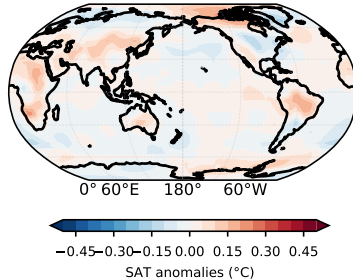
E \varepsilon = y - \hat{y}
