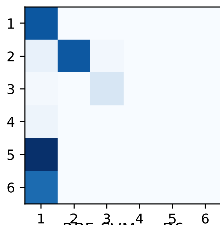
RBF-SVM 4 — B6 5
