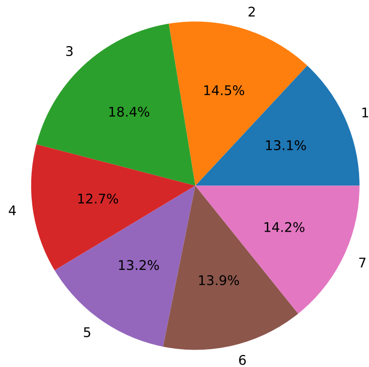
RDA
