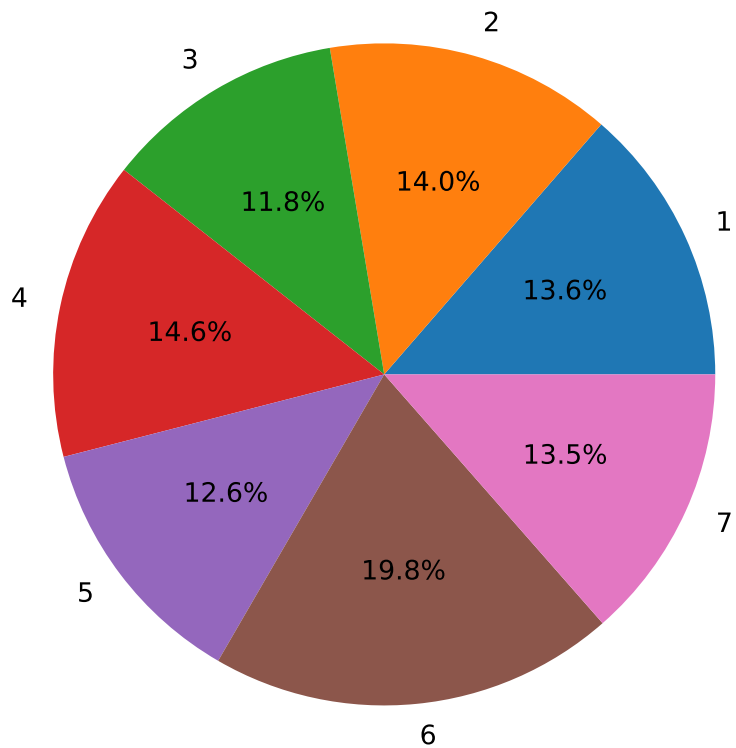
KNN
