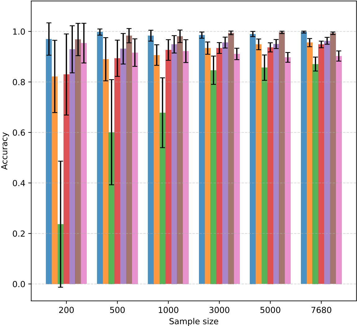
KNN
