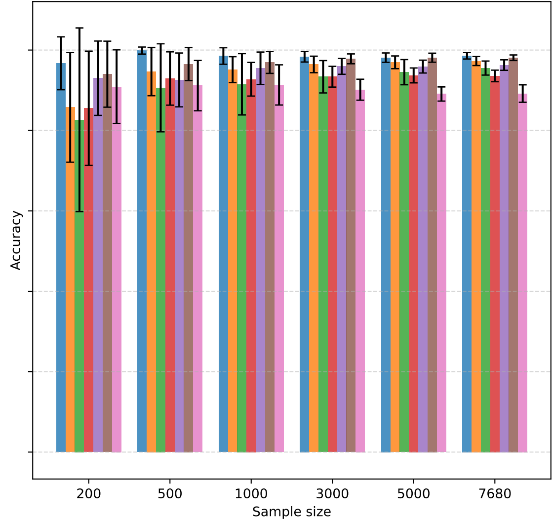
RDA
