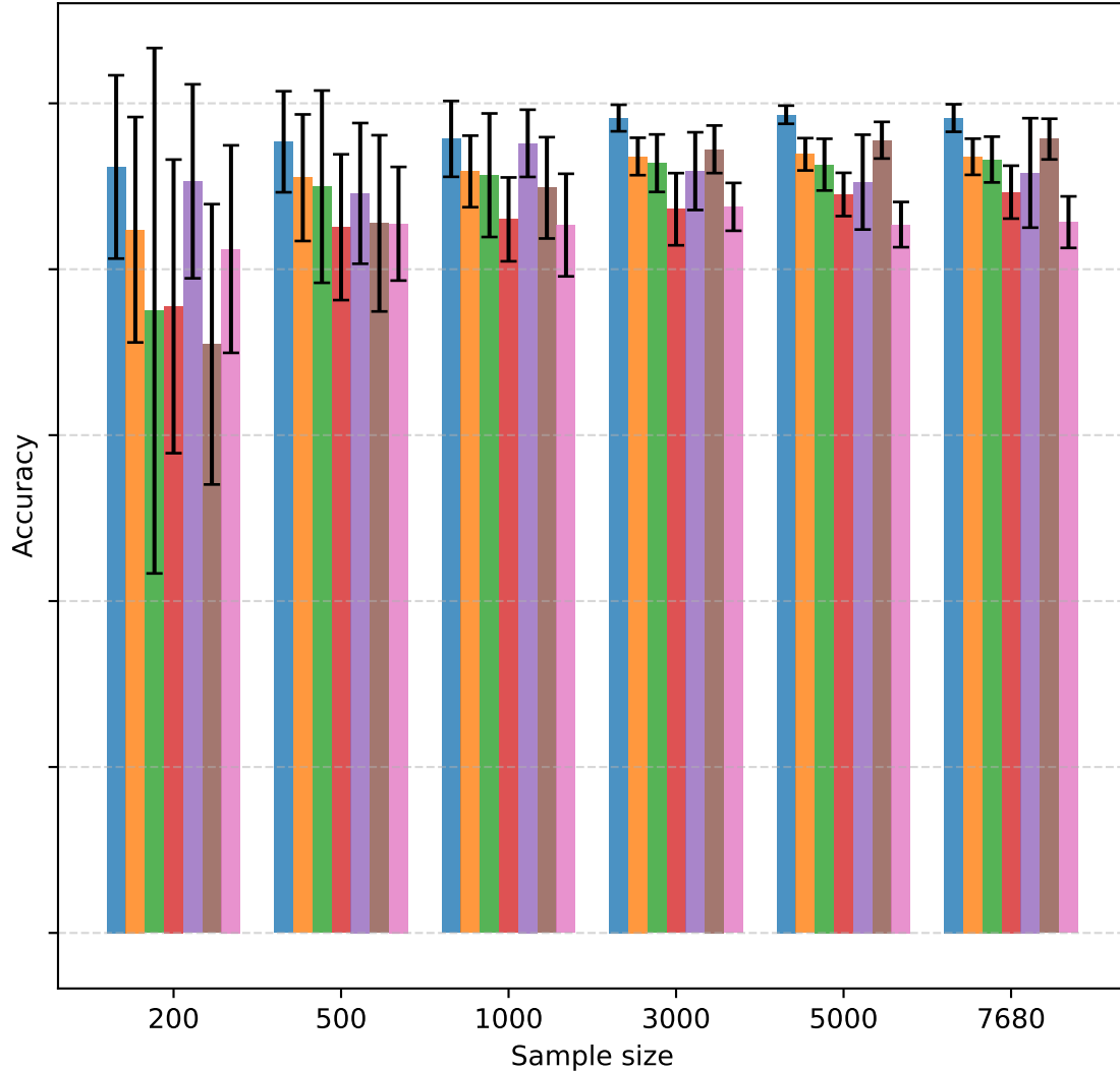
LogReg
