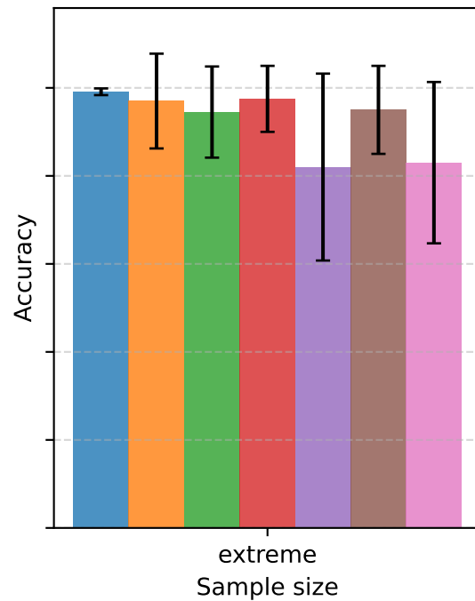
RDA
