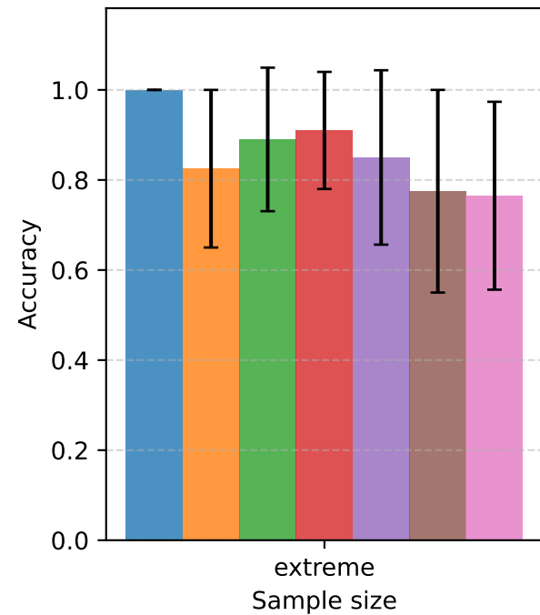
KNN
