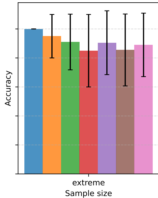
Hierarchy
