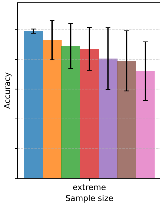
LogReg
