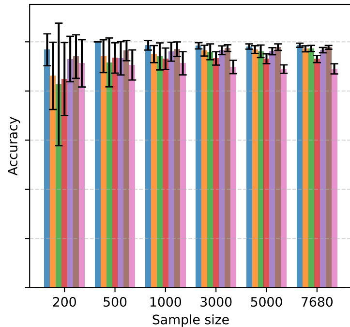
RDA
