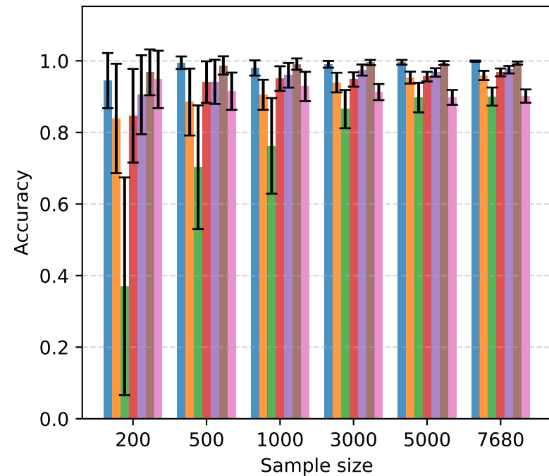
KNN
