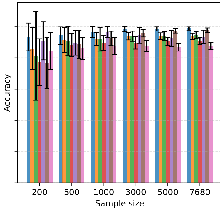
LogReg
