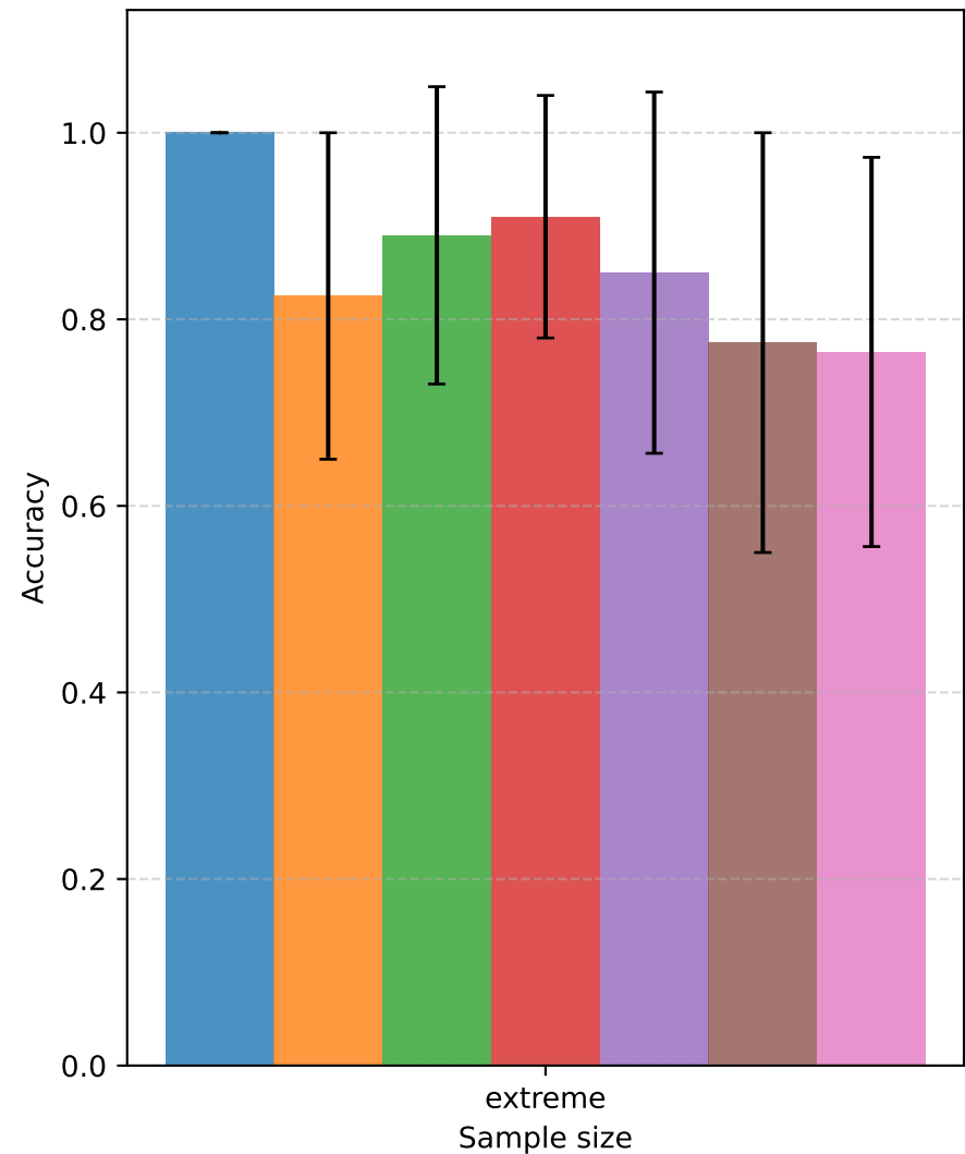
KNN
