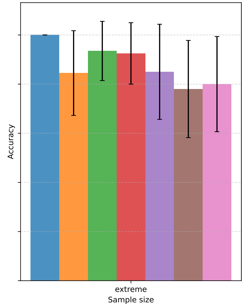
Hierarchy
