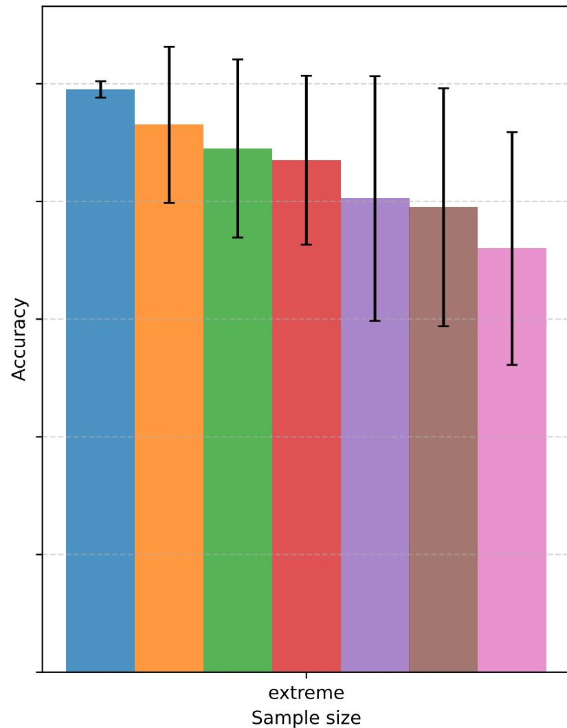
LogReg
