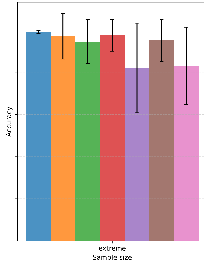
RDA
